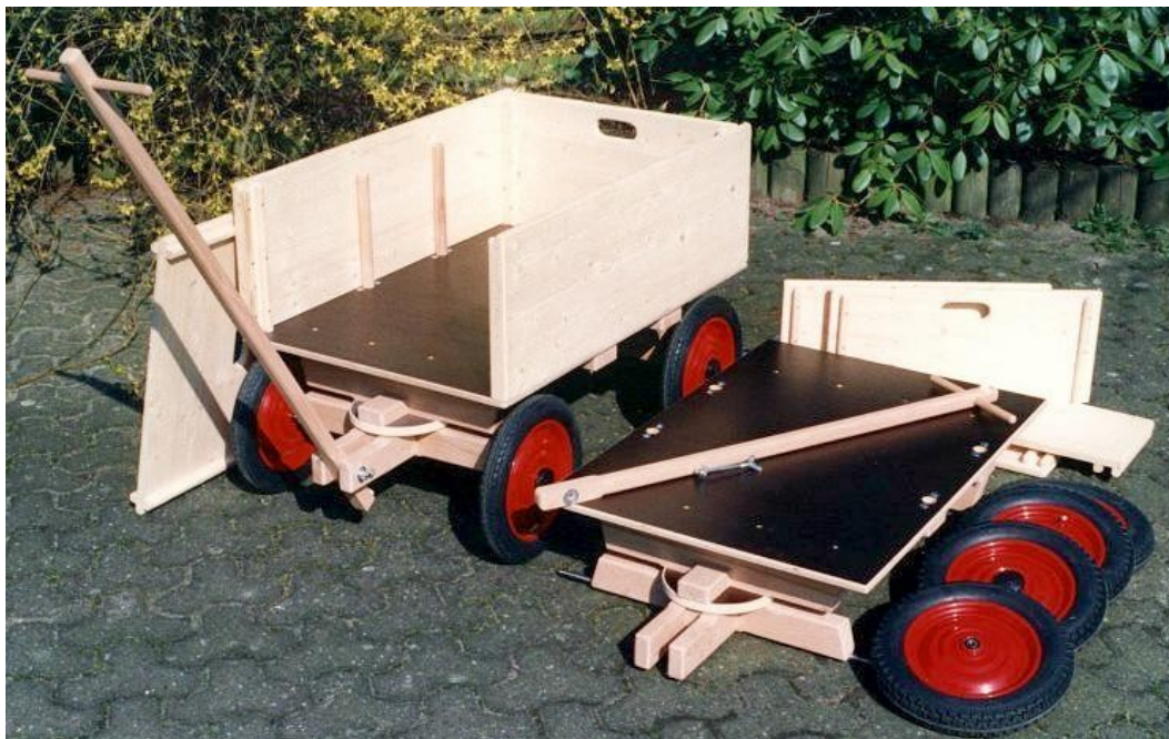
▲ 2 x DKZ 30/90 SV, links mit Rad Nr. 6, rechts mit Rad Nr. 3, zerlegt. Beide Wagen ohne Lackierung.
