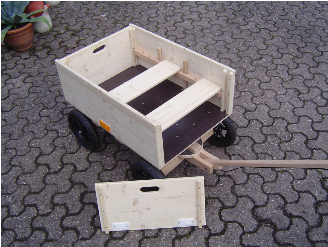
▲ DKZ 30/90 SV, mit Bremse, Sicherheits-Reflektoren und mit Sitzbank Typ: SBM mit 5 Sitzpositionen, ohne Lackierung.
